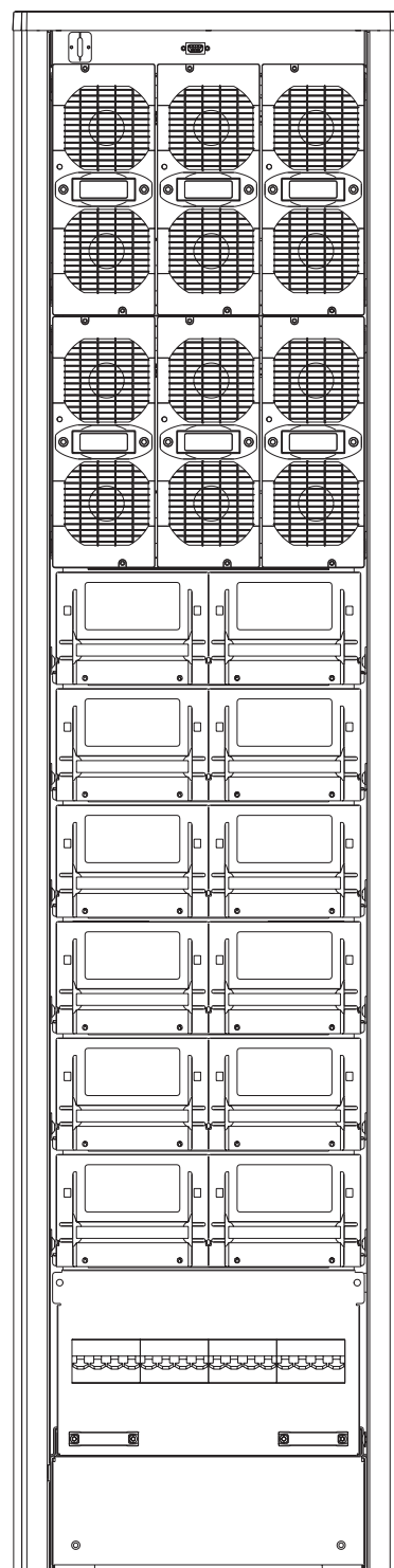
UPS Trimod® 20 - 6 slot UPS Trimod® 30TT con batterie interne
