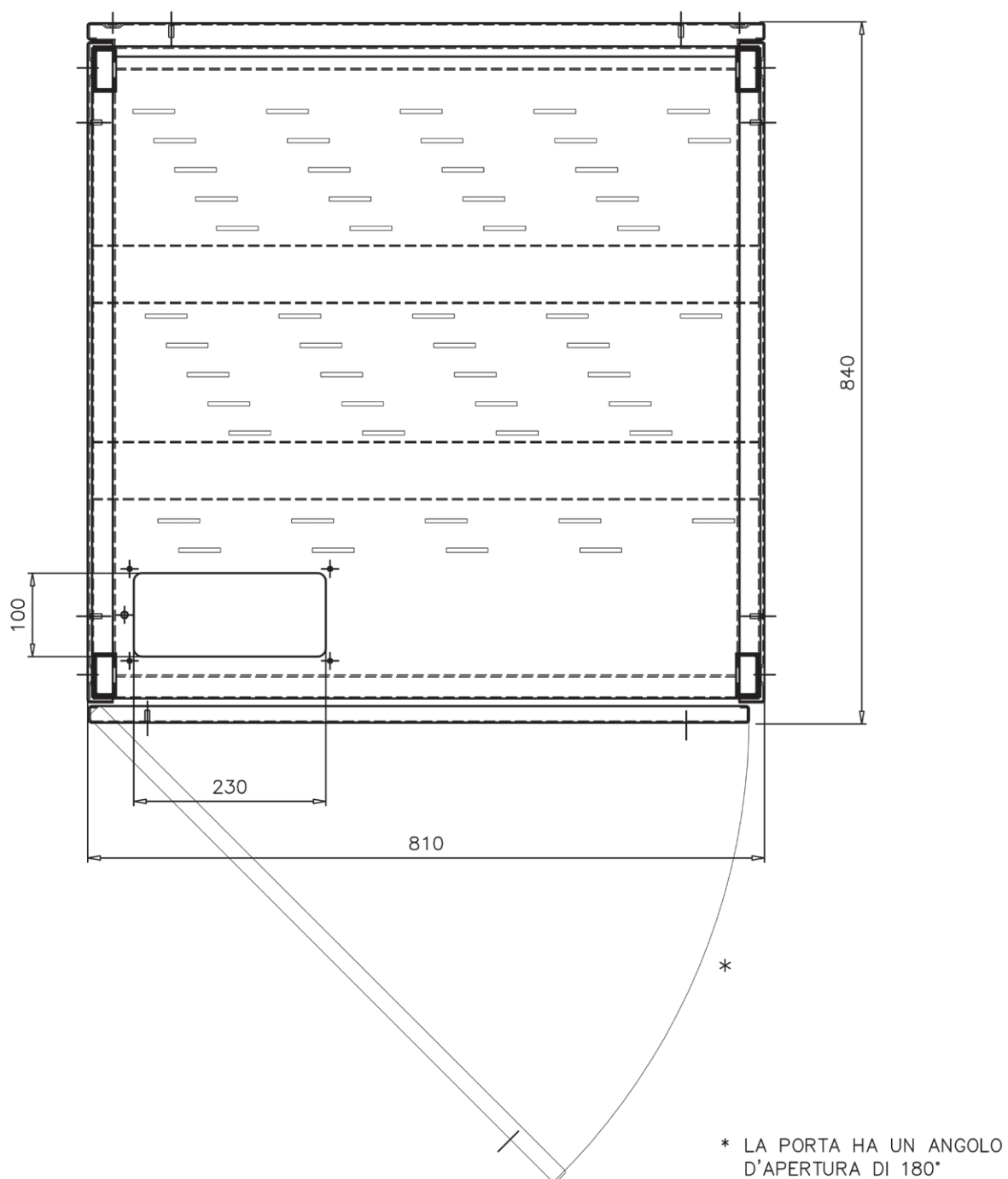
Vano connessioni elettriche armadio 810 x 840 x 1900
