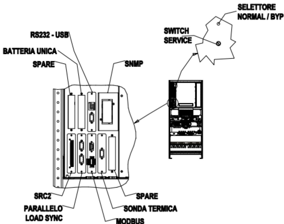
Figura 10 – Posizione schede di interfaccia KEOR HPE 200-250-300kVA
