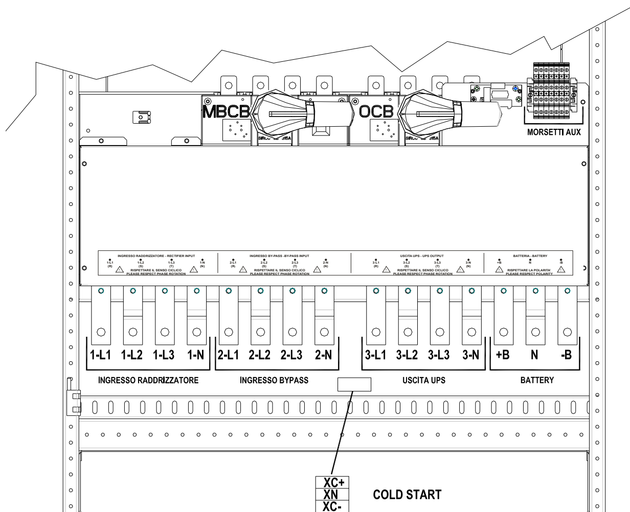
Figura 8A – Morsettiere KEOR HPE 200-250 kVA
