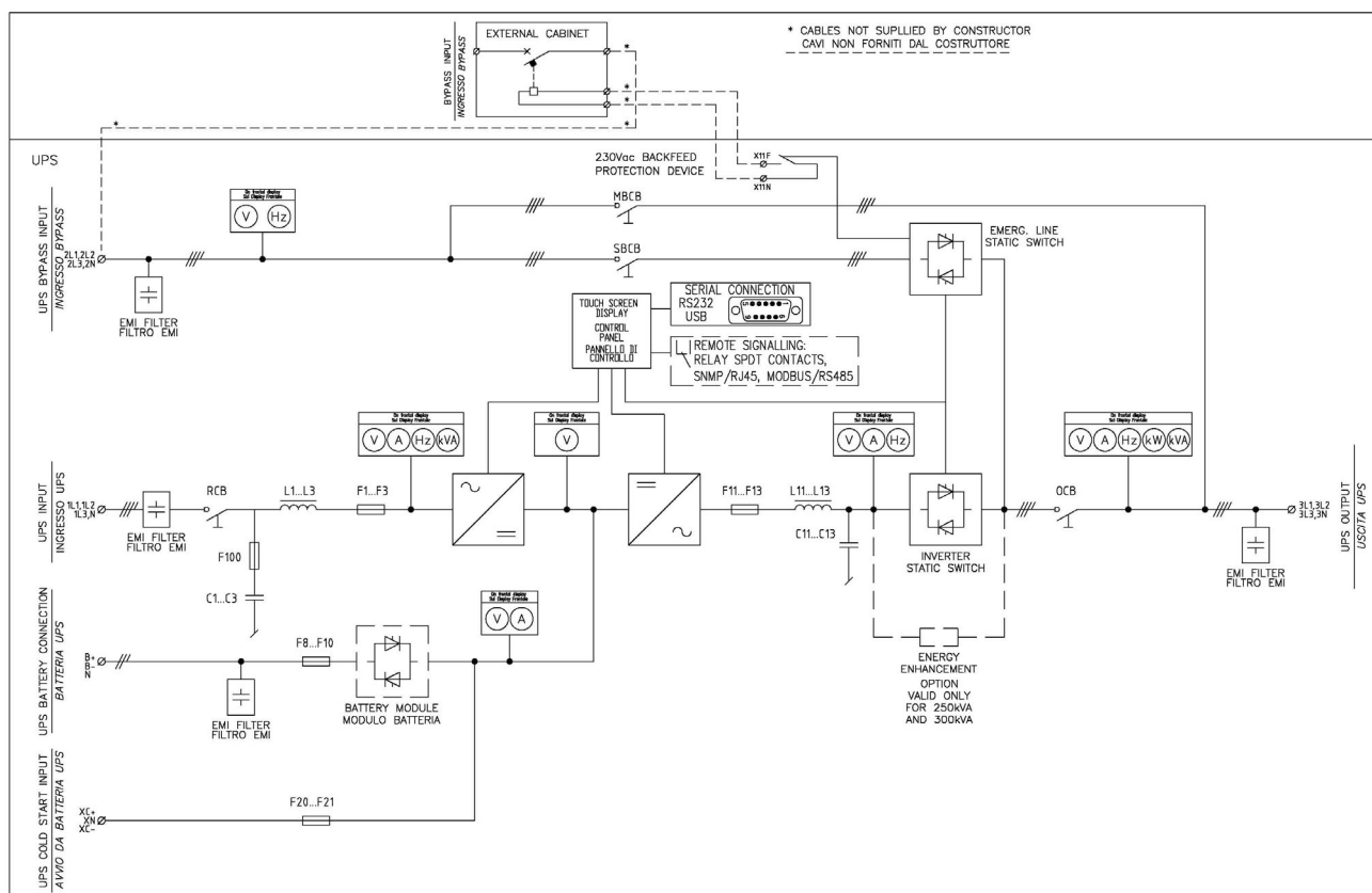
Figura 8 – Schema unifilare KEOR HPE 200-250-300kVA con collegamento al dispositivo esterno
