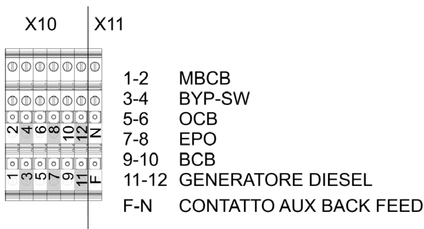
Illustration 9 – Bornes auxiliaires du KEOR HPE 200-250-300 kVA
