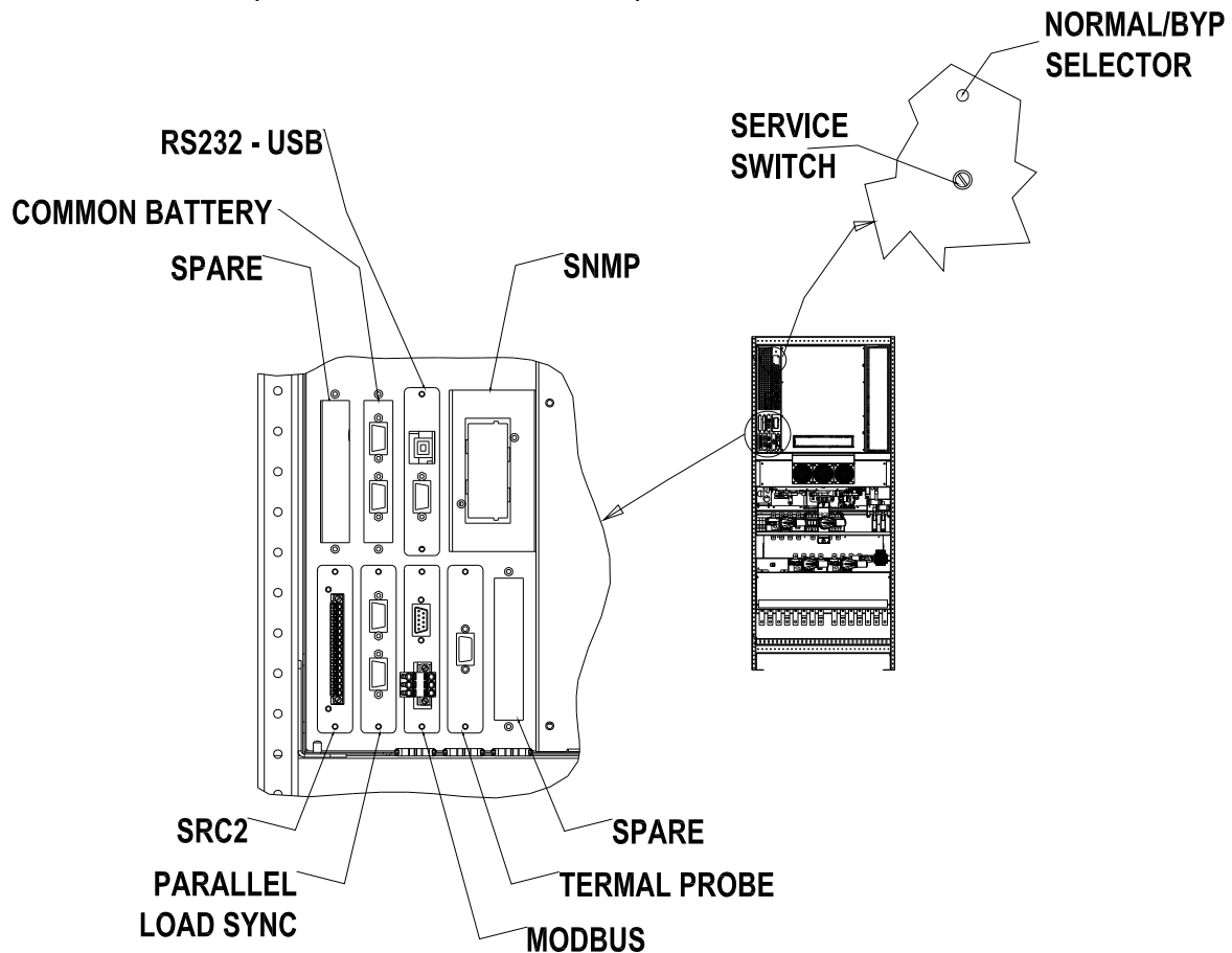
Illustration 10 – Position des interfaces de série du KEORHPE 200-250-300 kVA
