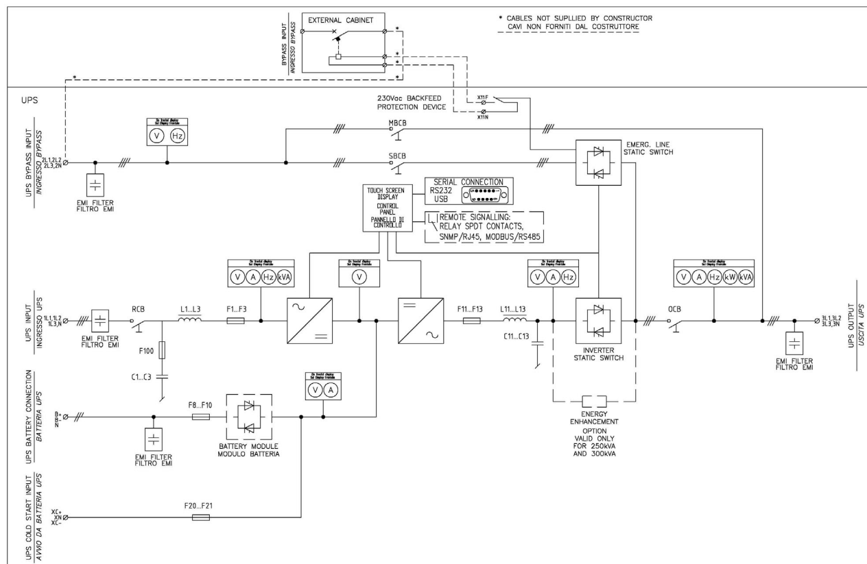
Illustration 8 – Diagramme à une ligne KEOR HPE 200-250-300kVA avec connexion à un périphérique externe
