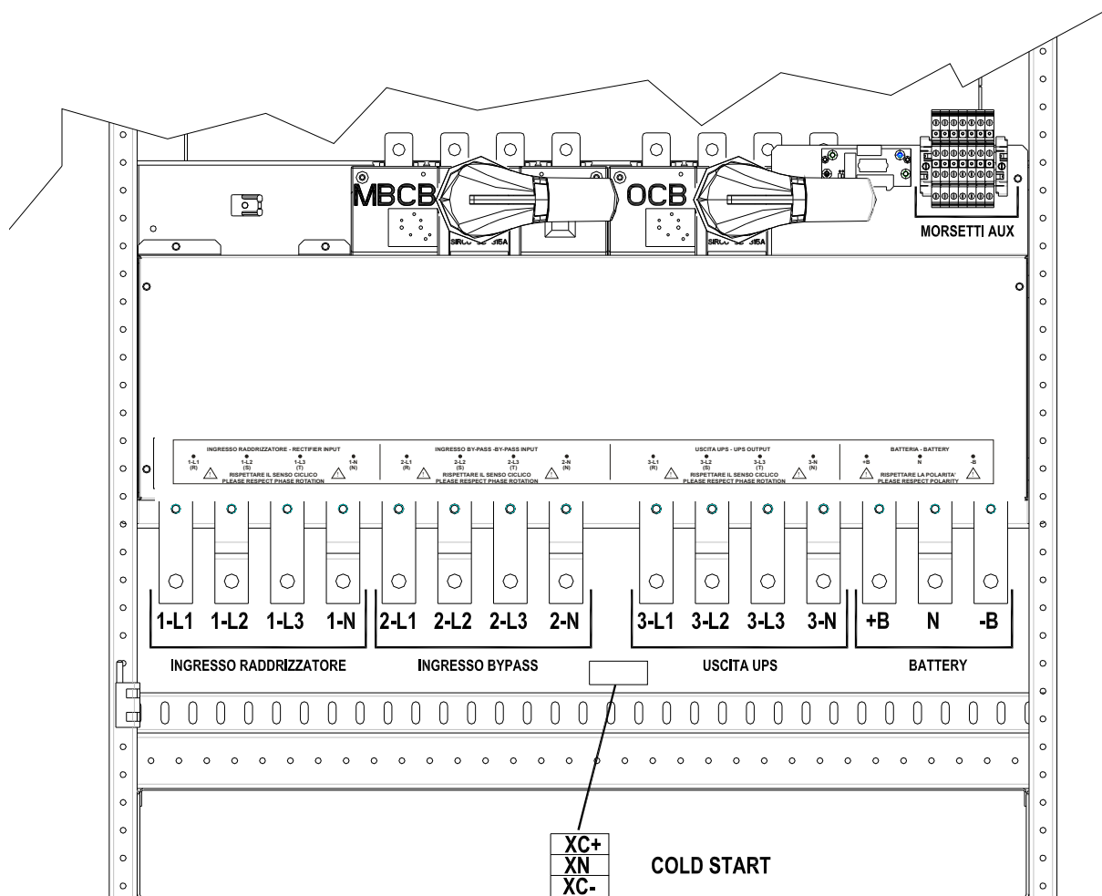
Figura 8B – Morsettiera KEOR HPE 300 kVA
