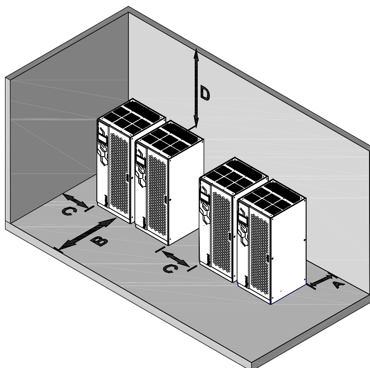
Illustration 5 – Dégagement minimum
