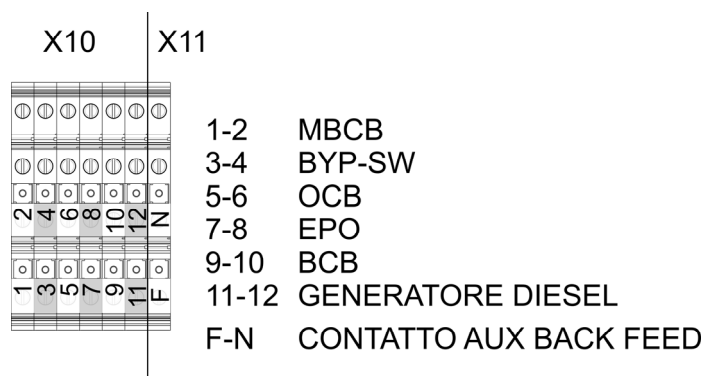
Figura 9 – Morsetti ausiliari KEOR HPE 200-250-300 kVA
